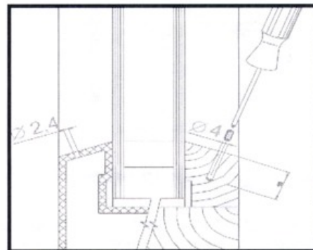
Obr.3 navrtáme otvory pro spodní upevnění fixace (pro plast ø 2,4 mm, pro dřevo ø 4 mm) Do otvoru 4 mm vešroubujeme fixační šrouby.
