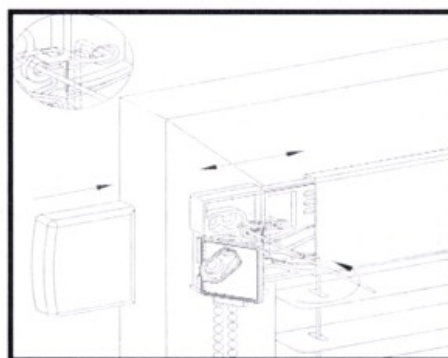
Obr.5 struny napneme přes horní koncovky, zajistíme kolíky, přebytečné struny zkrátíme a nasadíme krytky.
