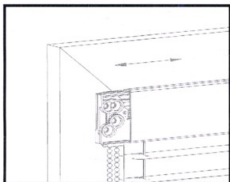
Obr.1 Posunutím koncovek nastavíme polohu montážních otvorů.
