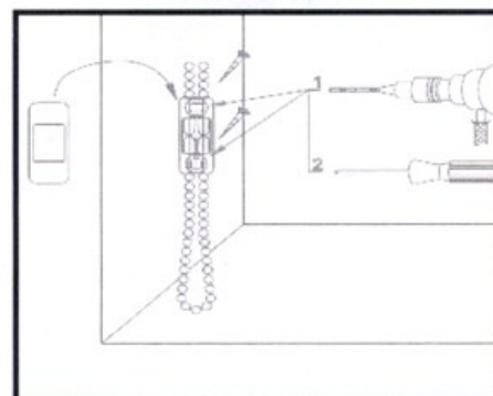
Obr.6 na straně ovládání přišroubujeme aretaci řetízku a nacvakneme krytku.
