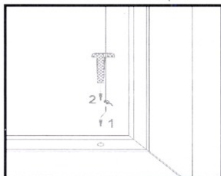
Obr.4 fixační struny s uzlíky vsuneme do otvoru, zajistíme kolíkem a struny potáhneme nahoru.
